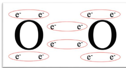
Figura 3: Emparelhamento de elétrons de do oxigênio molecular ( O_2 ).
