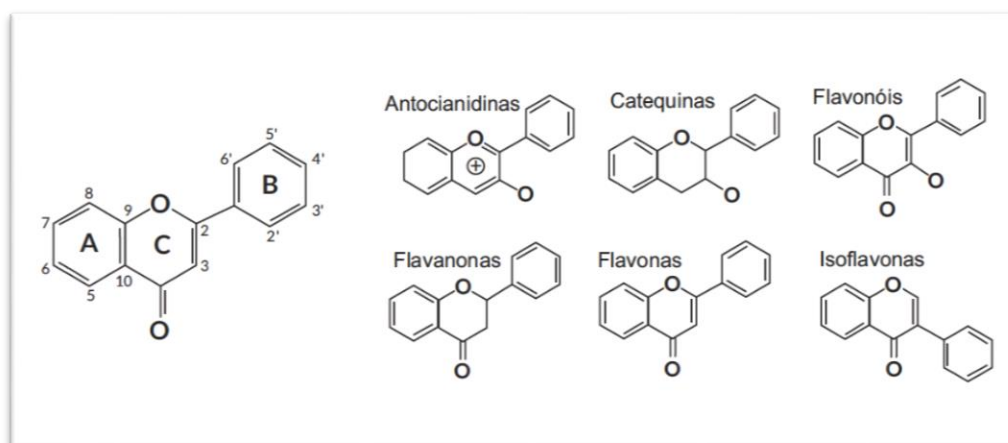
Figura 6: Estrutura química dos principais flavonoides
